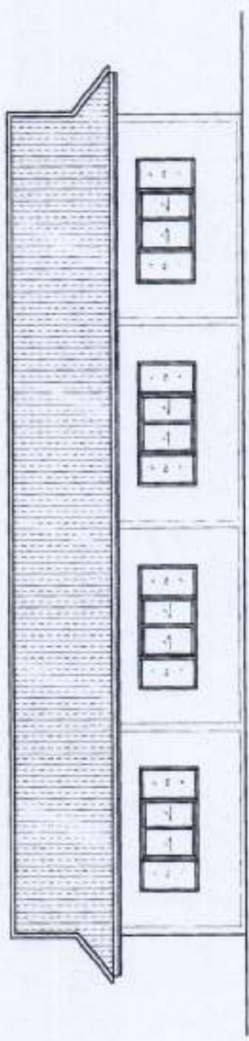
รูปด้าน - 3 มหานคร 1/75
